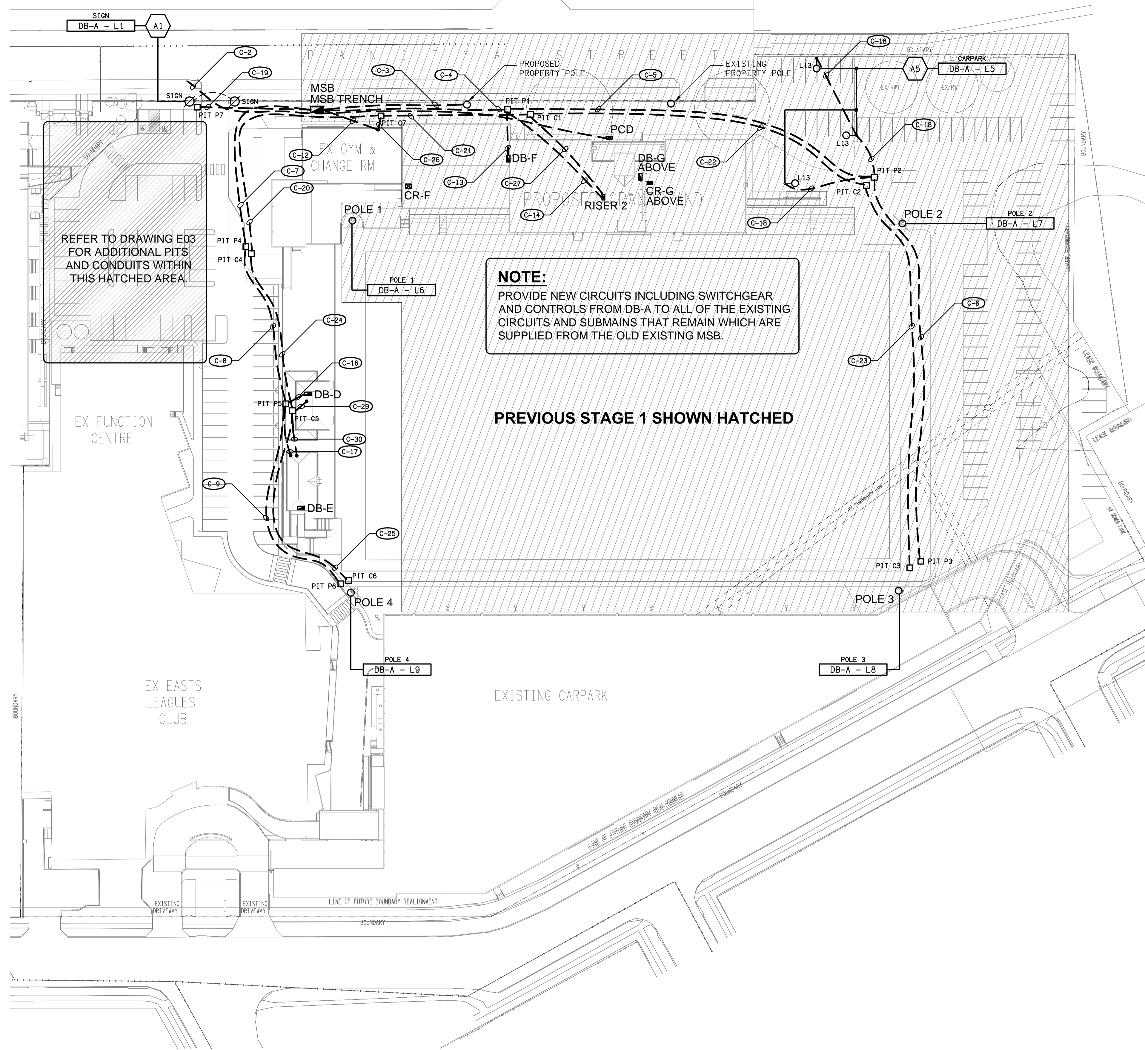
SITE PLAN PIT & CONDUIT LAYOUT SCALE 1: 500
